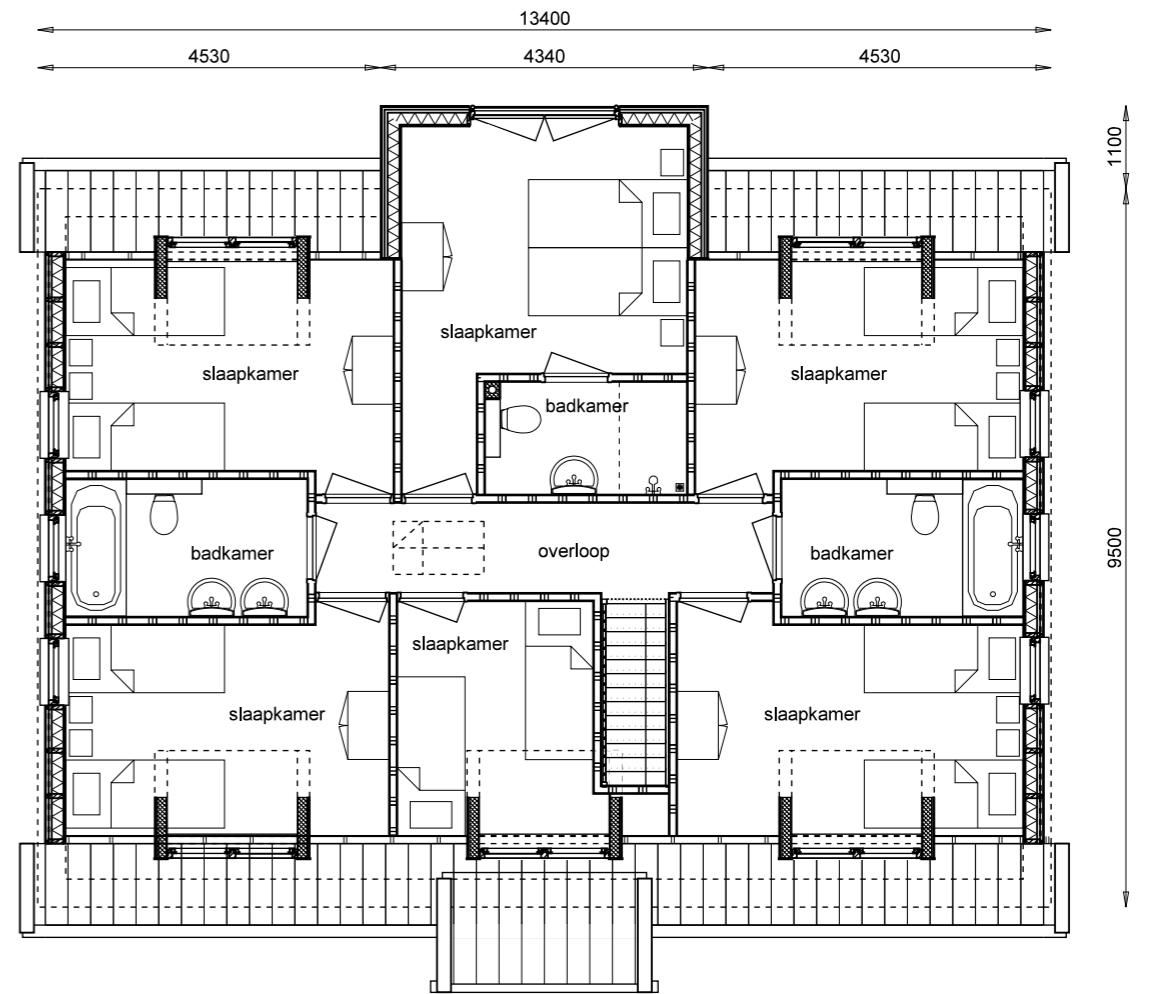
verdieping
