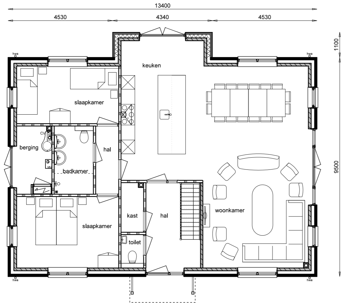
begane grond
